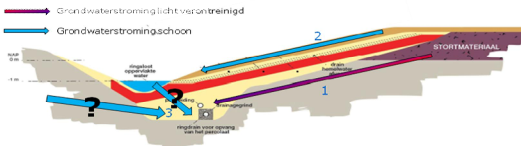
Figuur 6: Grondwaterstroming zijafdichting 2015
