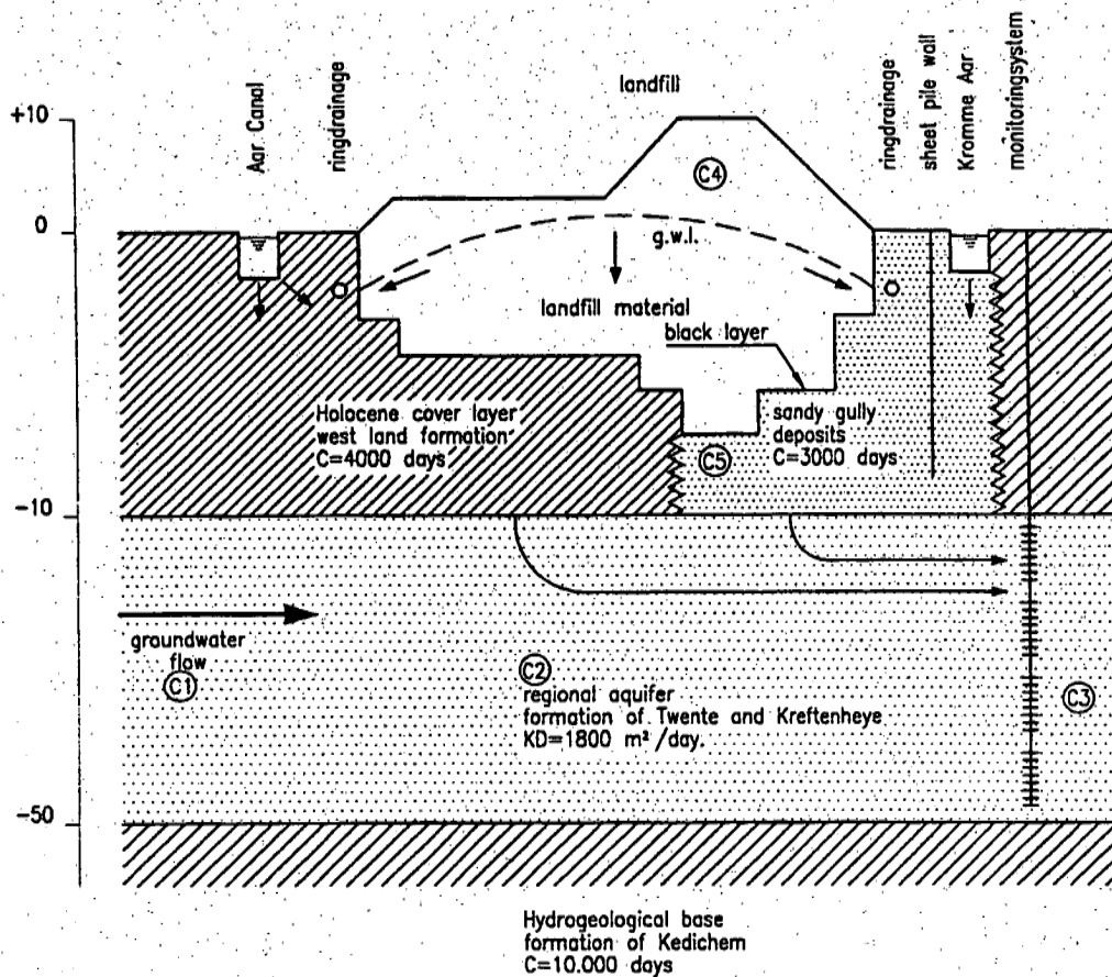
Fig. 7. Schematische bodemopbouw.
