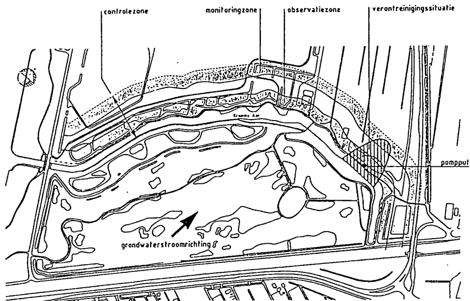
Beheersscenario met 1 pompput (bouwsteen 19a)
