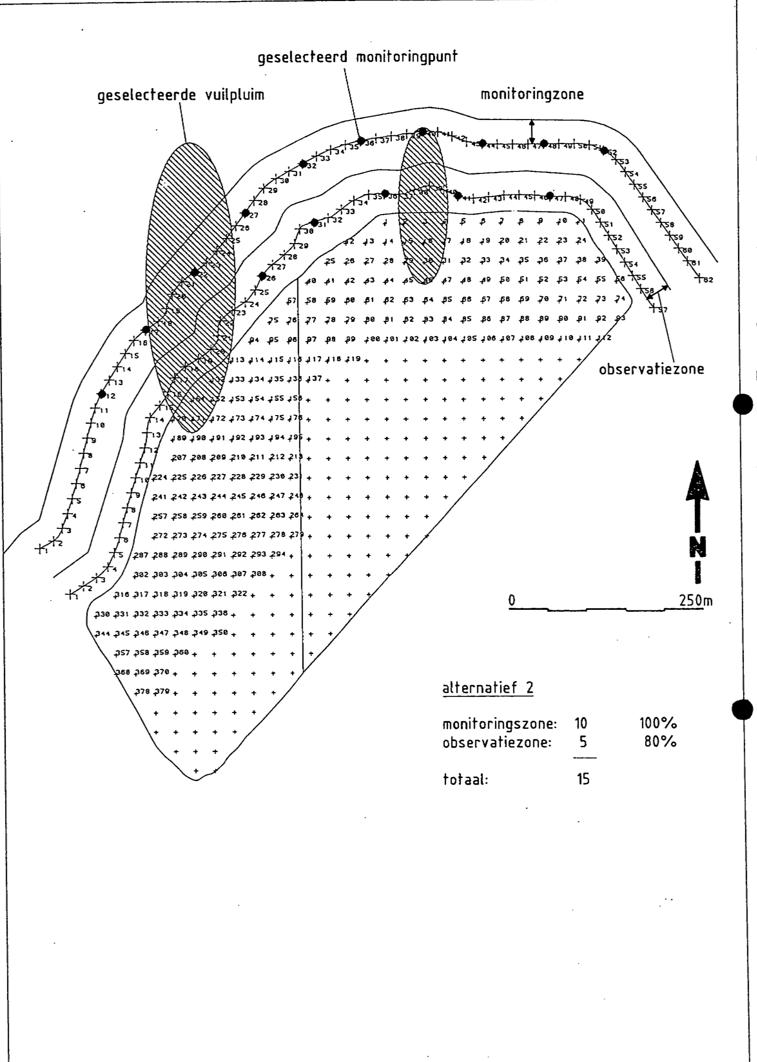
Fig. 8. Lay-out alternatief 2 monitoringsysteem
