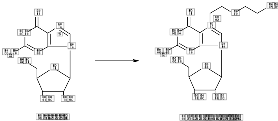
Abb. 9. Reaktion von S-Lost mit Guanosin.
