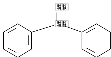
Abb.3. Strukturformel des Diphenylarsinchlorid (Clark I).
