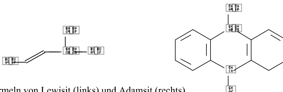
Abb. 6. Strukturformeln von Lewisit (links) und Adamsit (rechts).
