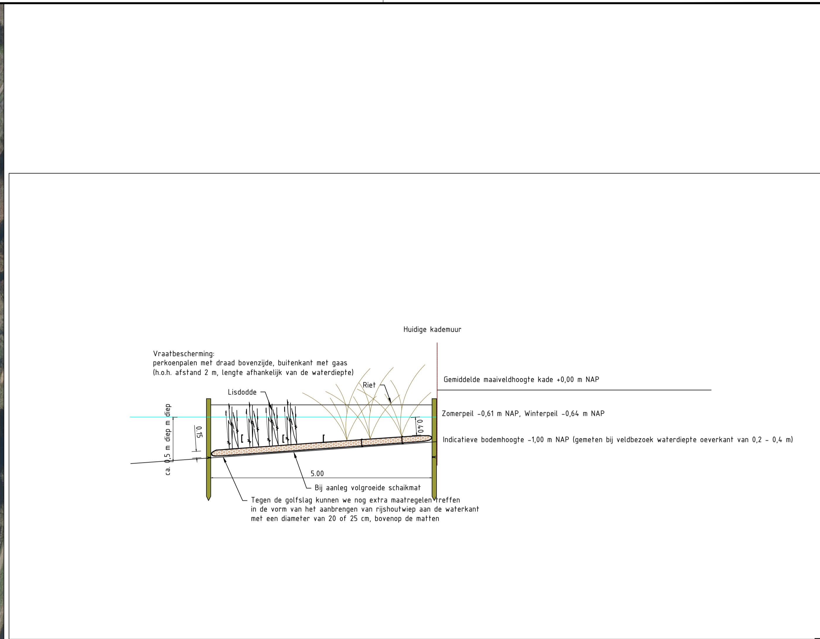
DOORSNEDE NVO Schaal 1:50
