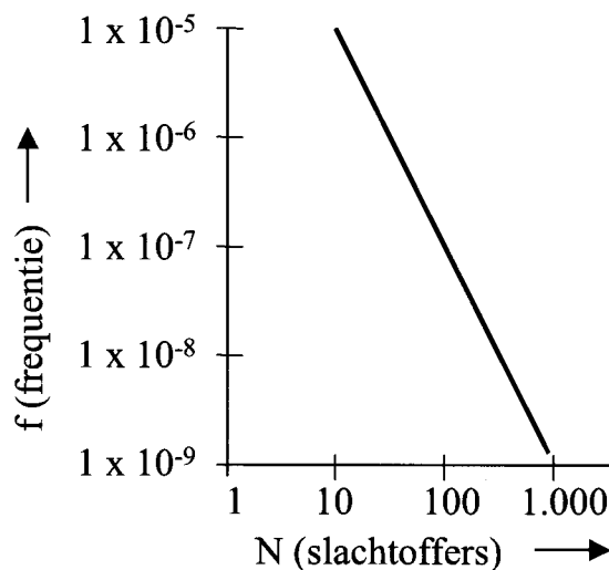
Figuur 1: Oriënterende waarde voor het groepsrisico volgens BEVI.
