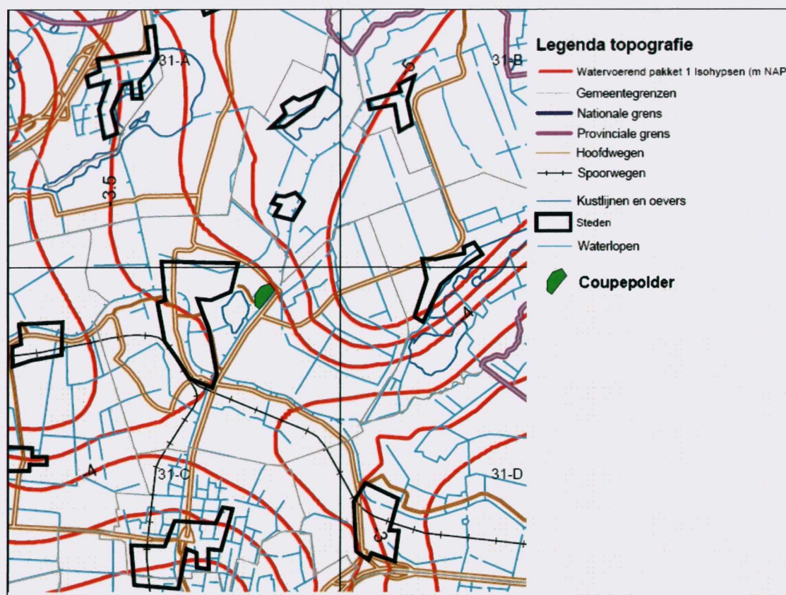
Figuur 2.3 Uitsnede uit berekend isohypsenpatroon eerste watervoerend pakket omgeving Alphen aan den Rijn, situatie april 1995 (TNO, 2002).
