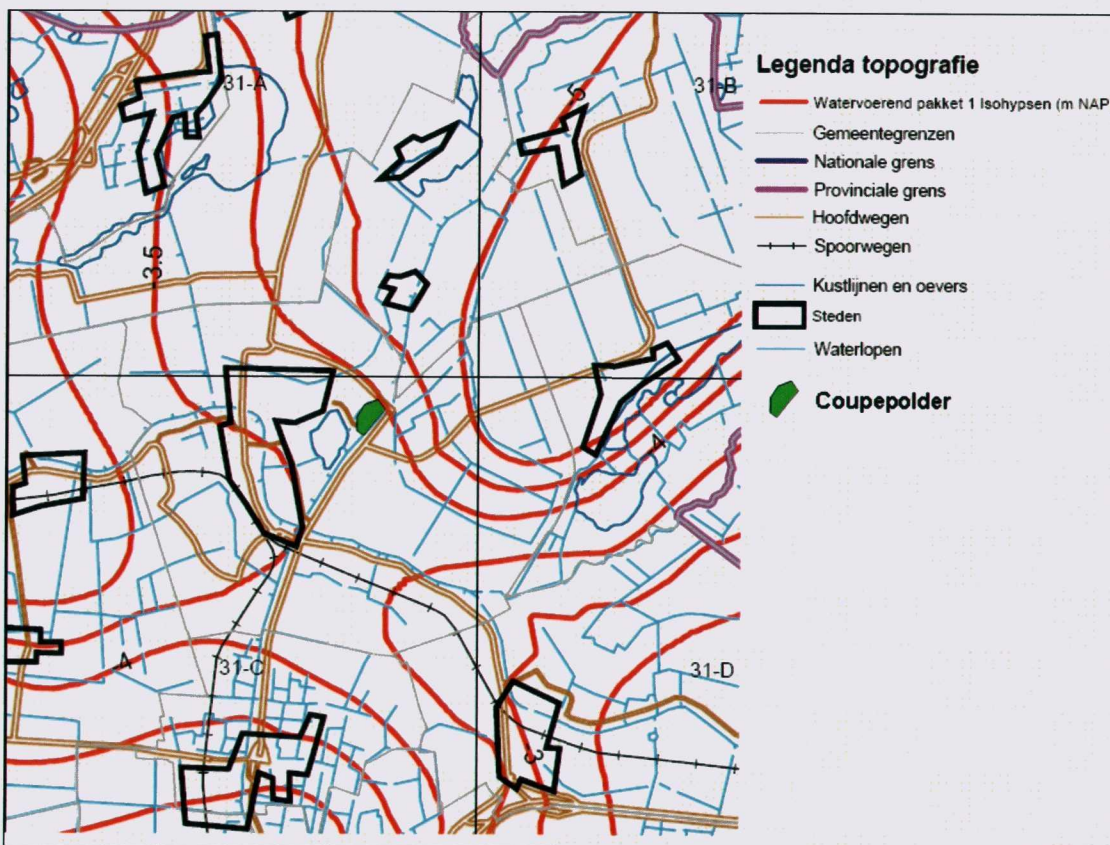
Figuur 2: Uitsnede uit berekend isohypsenpatroon eerste watervoerend pakket omgeving Alphen a/d Rijn, situatie april 1995 (TNO, 2002).
