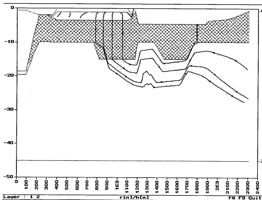
Fig. 5. Doorsnede zuid-noord van de stortplaats bekeken in westelijke richting met stroomlijnen die starten in het stortlichaam. De afstand tussen de markeringen op de stroombanen is 10 jaar.
