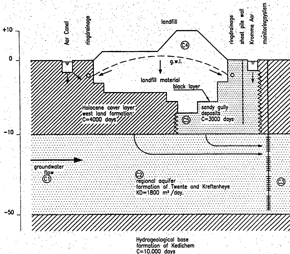
Fig. 7. Schematische bodemopbouw.
