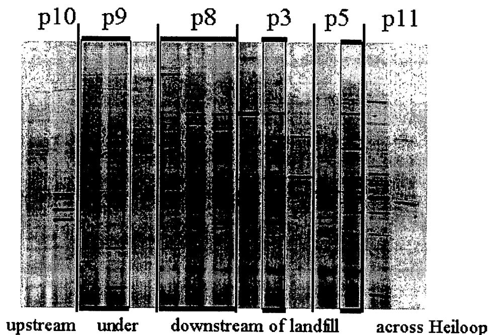
Fig. 10. DGGE profiel (40-60%) van grondwatermonsters van stortplaats Banisveld in september 1998. Monsters zijn weergegeven in de richting van de grondwaterstroming (links naar rechts). 1. p10f1; 2. P10f2; 3. P9f1; 4. P9f2; 5. P9f3; 6. P8f1; 7. P8f2; 8. P8f3, 9. P3f1; 10. P3f2; 11. P3f3; 12. P5f1; 13. P5f2; 14. P11f1; 15. P11f2.
