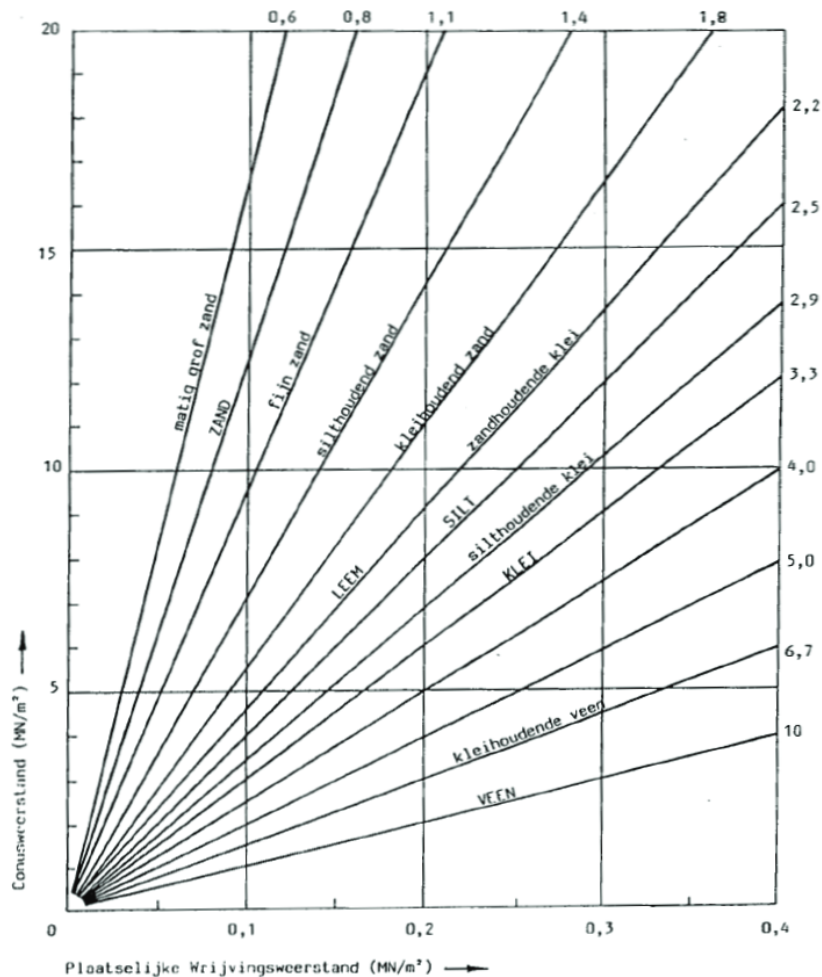
Figuur B2.1 Indeling grondsoorten op basis van conus- en wrijvingsweerstand
