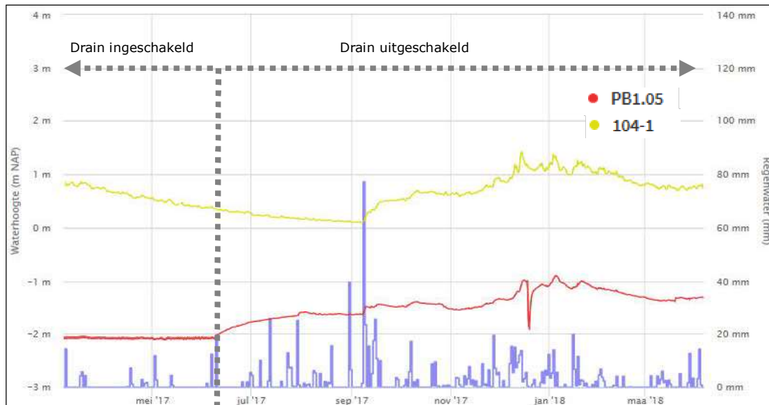
Figuur 16: Verloop grondwaterstanden in de stort nabij de ringdrain (PB1.05) en in de stort op 70 m afstand van de drain (104-1). In de figuur is op de rechter as de neerslag opgenomen.
